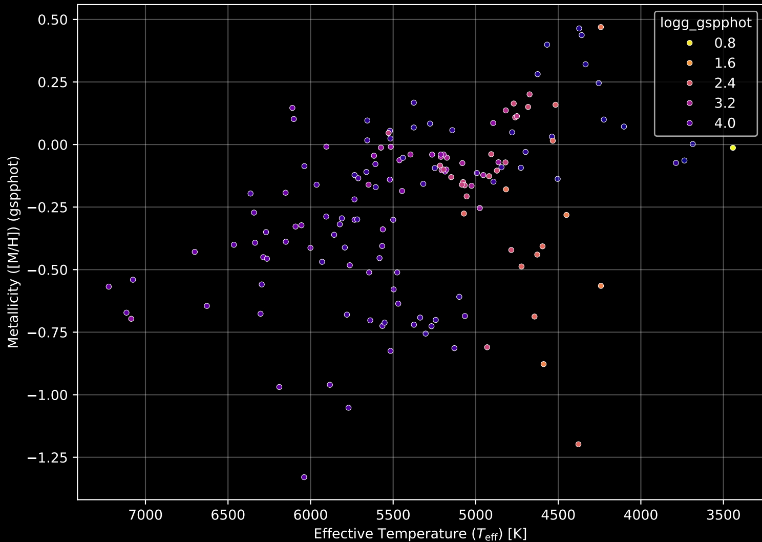
APOGEE DR17 Field: [284-36-O_TESS] Stellar Population Parameters (n= 151)
